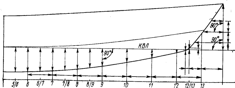
Рис. 99. Теоретический чертеж контура днища (проекция «бок») носовой части яхты «Гаранга».
