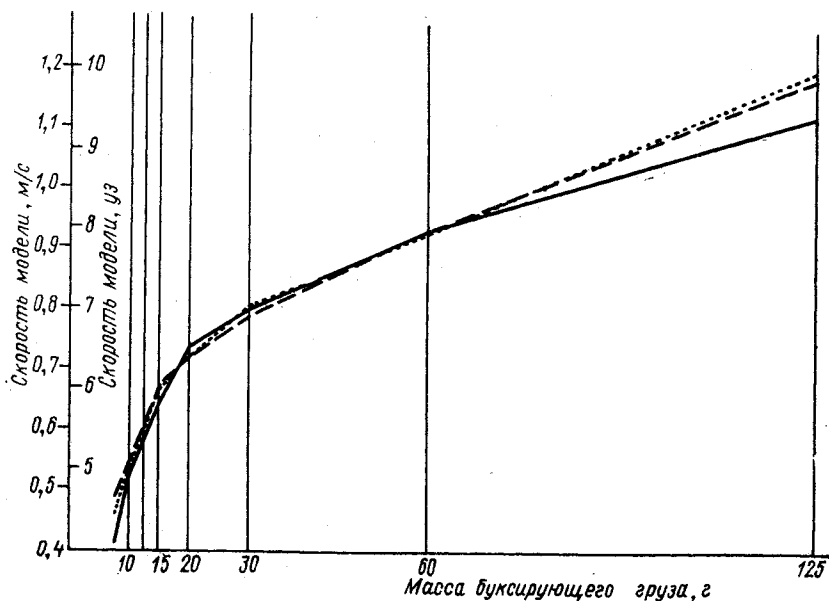
Рис. 3. Результаты буксировочных испытаний моделей (зависимости скорости от массы буксирующего груза) для трех различных килевых яхт — однотонокников, свидетельствующие о высокой точности примененного метода.
