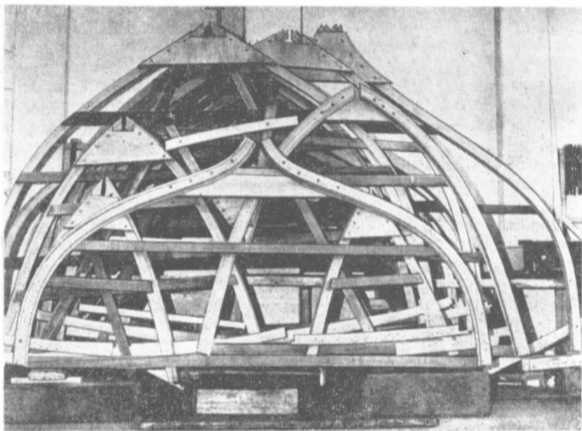
Рис. 63. Ламинированные шпангоуты не только прочнее, но лучше сохраняют приданную им форму, чем традиционные гнутые.
