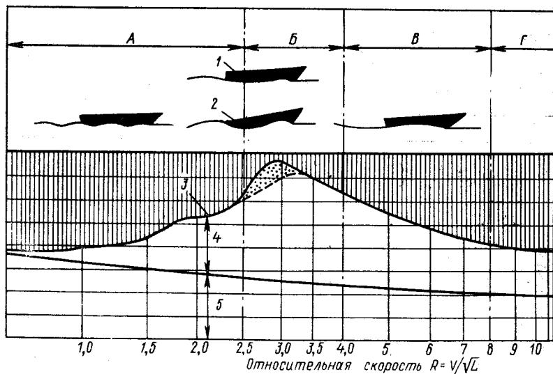
Рис. 7. Режимы движения яхты и зависимость сопротивления трения и формы от относительной скорости судна.
