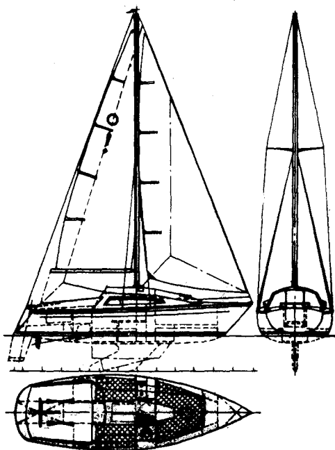
Рис. 28. Оснастка яхты «Таранга» — типичный вариант для туристской парусной яхты. Включая «автоматический» стаксель, имеются только три стакселя; спинакер не предусматривается.
