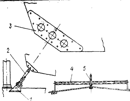
Рис. 168. «Автоматический» стаксель без рейки на яхте «Омега-S».
