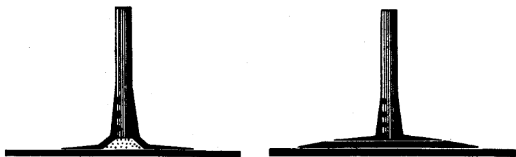
Рис. 136. Виды приформовки внутренних переборок из фанеры.
