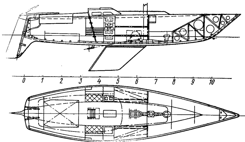
Рис. 48. Схема общего расположения яхты «Импробэйбл».
