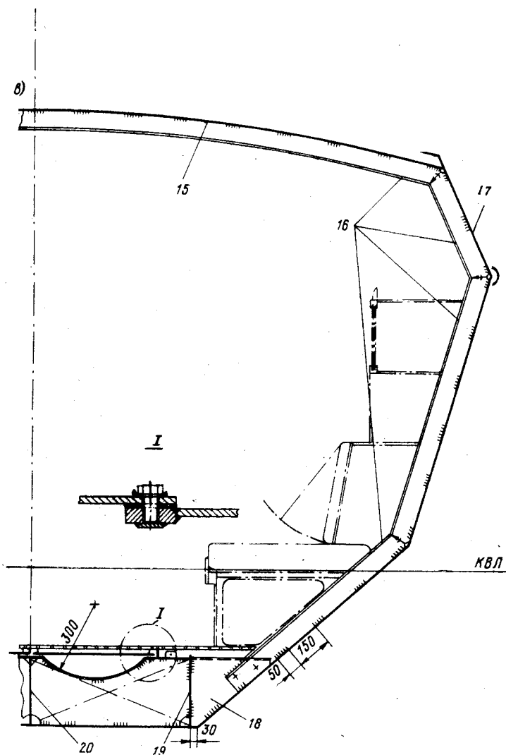
Рис. 4, в. Конструктивный «мидель-шпангоут» стальной яхты «Гидра»: в — рамный шпангоут — шп. 10.
