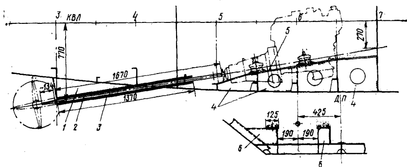
Рис. 107. Линия вала и фундамент под двигатель на яхте «Гидра» (установка двухвальная).
