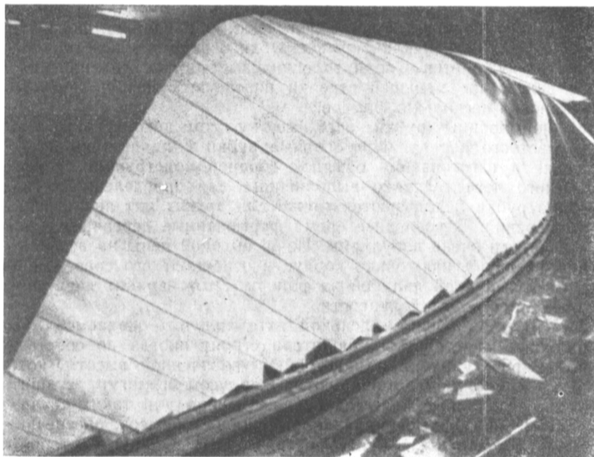
Рис. 79. Подогнанные и прихваченные скобками листы шпона надо снимать по отдельности и после нанесения клея вновь укладывать на болван.
