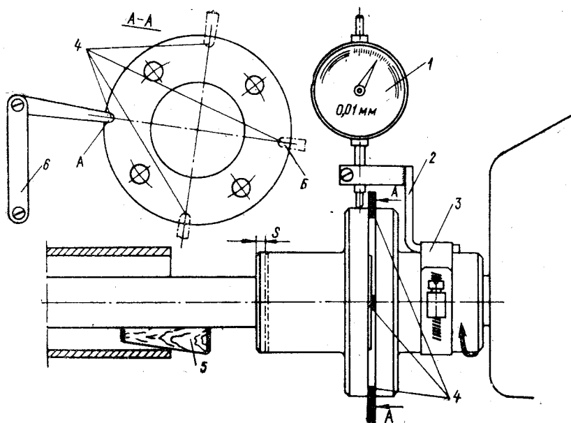
Рис. 178. Схема установки индикатора для контроля смещения линии вала и использования шнура для замера излома.
