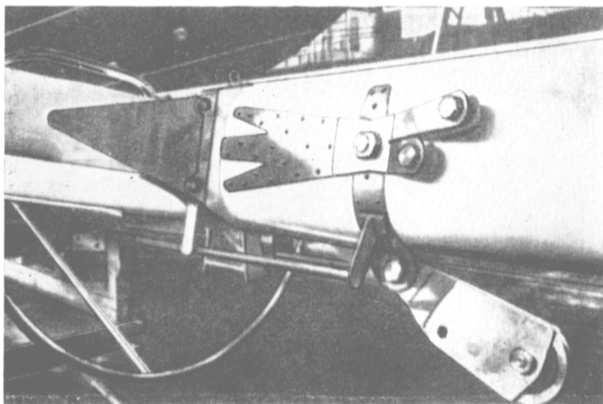
Рис. 161. Традиционный узел крепления нижних вант и краспиц на деревянной мачте моторно-парусной яхты.
