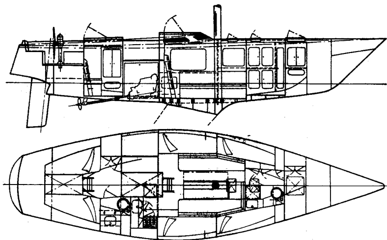
Рис. 32. Схема общего расположения яхты «Сланкер».
