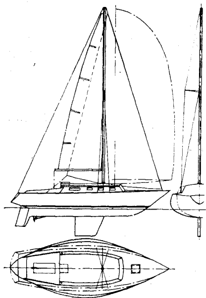
Рис. 23. Проект яхты, созданный по формуле IOR, воспринятый как чрезвычайный «выжиматель формулы» со сверхшироким корпусом.
