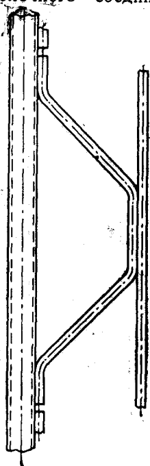
Рис. 112. Конструкция рамного шпангоута. Слева — для деревянной палубы, справа — для палубы из армоцемента.
