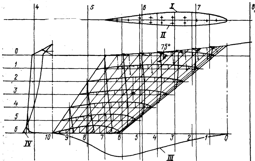
Рис. 15. Теоретический чертеж плавникового кия.
