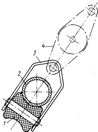
Рис. 158. Простой роликовый ползун на трубчатом погоне.
