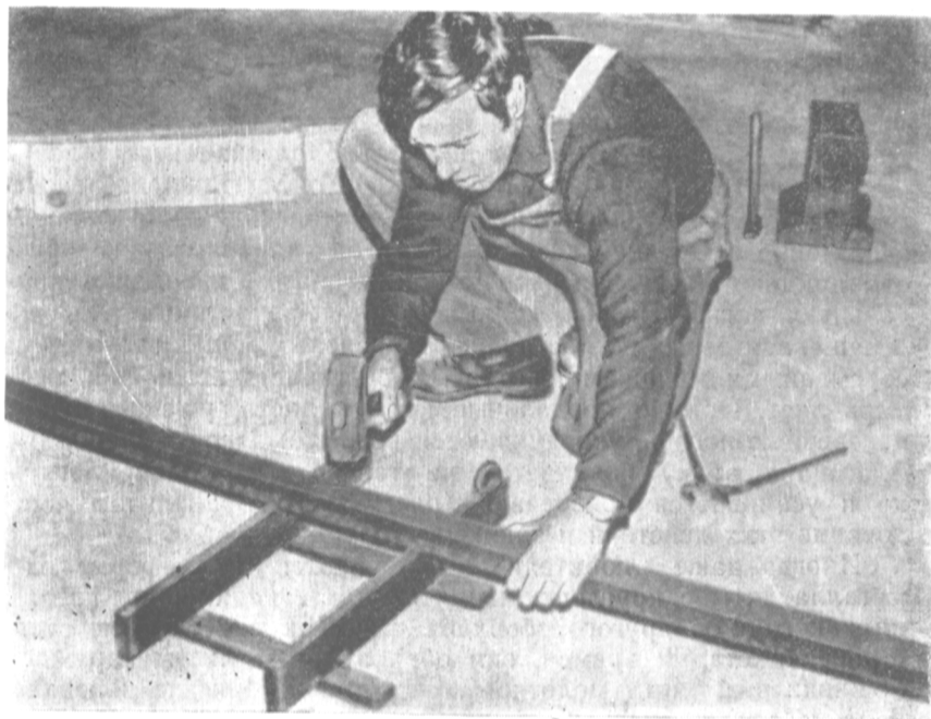
Рис. 85. Гибка профиля с помощью кувалды.
