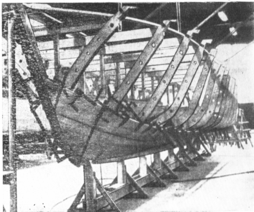
Рис. 69. При обшивке корпуса по поперечным шаблонам отдельные планки склеивают по пазам. К килю и форштевню планки крепят на шурупах.
