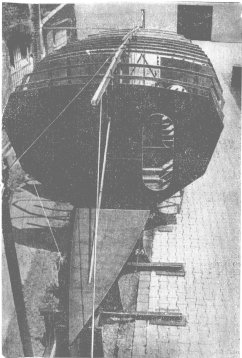
Рис. 103. Монтаж корпуса 14-метровой яхты «Гидра» начинается с установки жесткой переборки. После угловой точечной сварки к днищевому листу переборку выравнивают строго вертикально с помощью отвеса и закрепляют одной-двумя диагональными распорками. Верхняя прочная рейка служит временной опорой, по которой выверяют шпацию для всех других шпангоутных рам и переборок.
