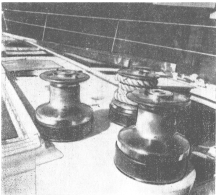
Рис. 163. Функциональное расположение шкотовых лебедок на палубе яхты «Христина».
