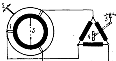
Рис. 200. Принцип телепередачи направления ветра на индикатор (сельсин).
