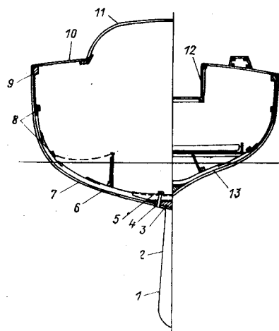
Рис. 49. Конструктивный мидель-шпангоут «Импробэйбл».
