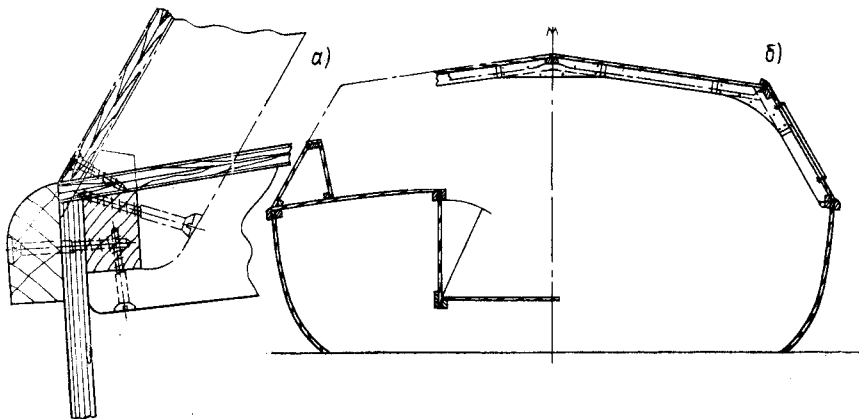
Рис. 81. Пример относительно простой конструкции корпуса с надстройкой — баком на яхте «Контра» длиной 6,80 м. Сечения в районе кокпита (а) и палубы (б). Конструкция всех соединений рассчитана так, что ни одна из кромок фанеры не остается открытой.
