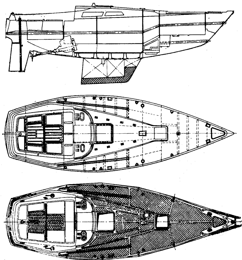
рис. 123. Конструктивный чертеж парусной яхты «Корнет-32»
