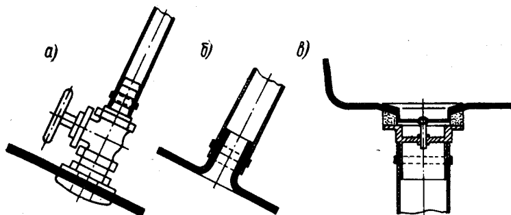
Рис. 133. Конструкции выводов трубопроводов через наружную обшивку.
