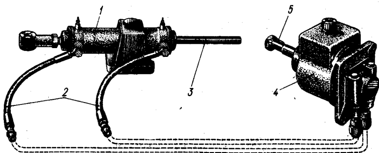
Рис. 142. Ручное гидравлическое рулевое устройство (50—1600 Н·м).
