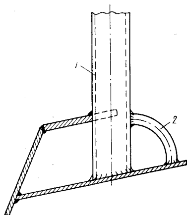
Рис. 156. Крепление леерной стойки на стальной яхте.
