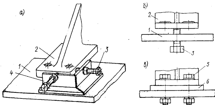
Рис. 179. Приспособление для перемещения двигателя при центровке: а — по горизонтали; б — по вертикали; в — постановка прокладок.
