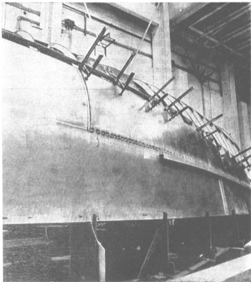
Рис. 88. Последовательность сварки при монтаже листа наружной обшивки: после того как стык сварен полностью и выровнен, прихватывают точечной сваркой продольный шов. На время сварки обшивку к набору временно прижимают струбцинами.
