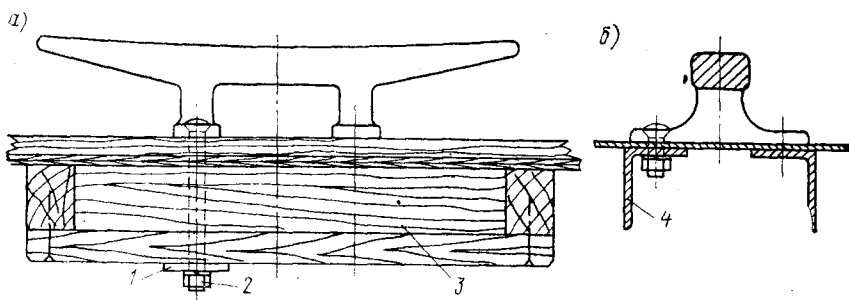
Рис. 155. Крепление утки к деревянной (а) и стальной (б) палубе. 1 — шайба 40×5; 2 — болт М10; 3 — деревянная подушка; 4 — угольник 50×40×5.
