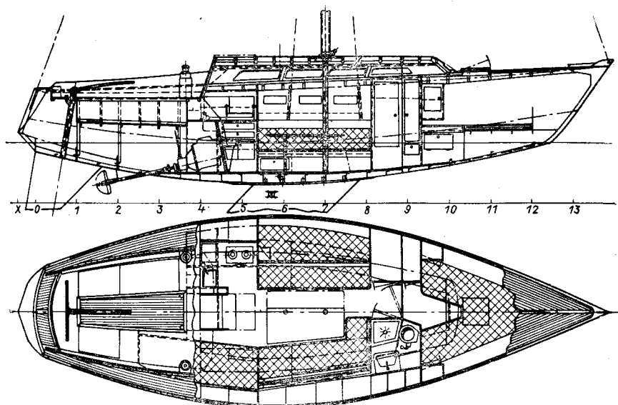
Рис. 27. Схема общего расположения яхты «Таранга» самостоятельной постройки.
