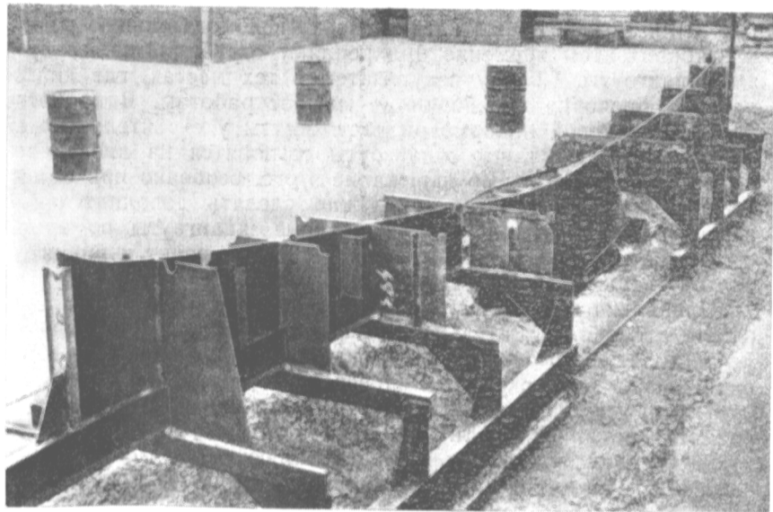
Рис. 102. Для постройки стапеля на неровном полу не обойтись без нескольких бетонных опор. В середине стапеля виден установленный киль, который на своем месте заменяет стапель.
