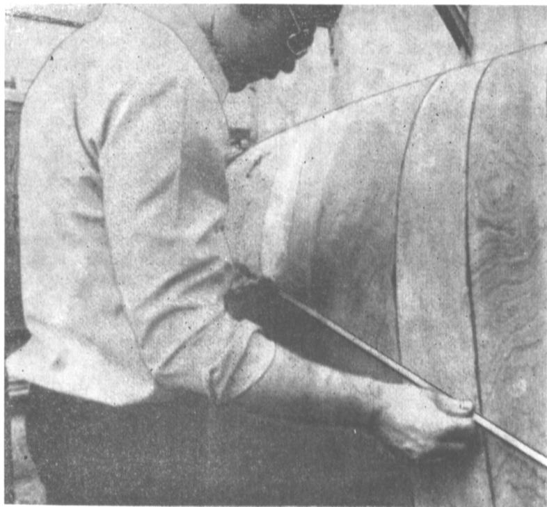
Рис. 77. Диагональная обшивка из полос фанеры на стапель-кондукторе.
