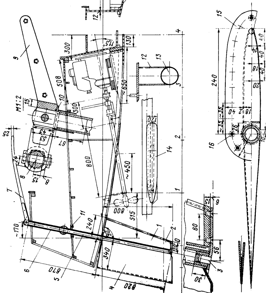
Рис. 82. Конструкция руля и дейдвуда гребного вала из нержавеющей стали для яхты длиной 7,5 м. Фундамент для снижения структурного шума изготовлен из дерева и имеет соединения из алюминиевых угольников.
