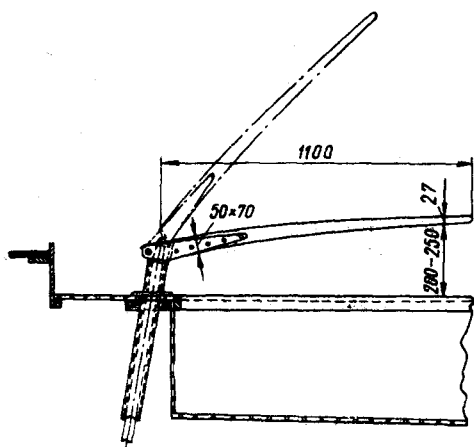
Рис. 140. Схема установки румпеля на 10-метровой яхте.
