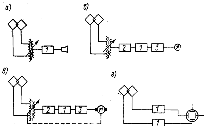
Рис. 187. Принципиальные схемы различных радиопеленгаторов с гониометром: а — с определением минимального пеленга на слух; б — с визуальным индикатором; в — с автоматическим индикатором; г — двухканальный радиопеленгатор с визуальным индикатором.
