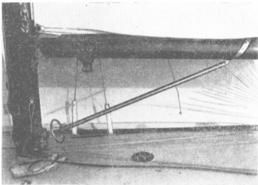
Рис. 164. Винтовая (шпindelная) оттяжка гика заменила на современных яхтах традиционные тали.
