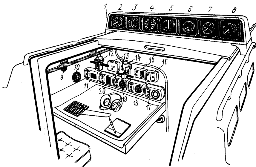
Рис. 198. Типовое расположение приборов на крейсерско-гоночной яхте.
