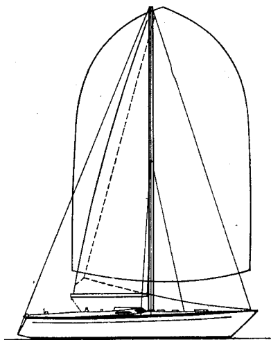
Рис. 31. Схема парусности яхты «Спанкер».
