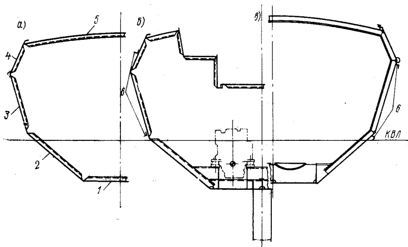
Рис. 96. «Мидель-шпангоут» яхты «Гидра» упрощенной конструкции: а — промежуточный шпангоут; б — сечение по кокпиту; в — рамный шпангоут. 1 — днищевой лист обшивки; 2 — скуловой пояс; 3 — ширетрек (фортвой пояс); 4 — комингс бака; 5 — палуба; 6 — монтажные ребра жесткости из угольника.
