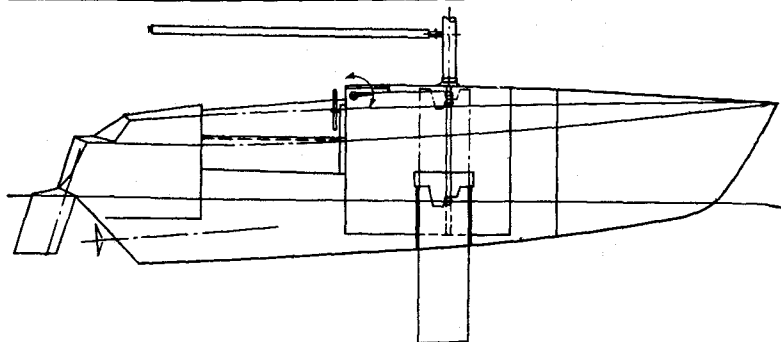
Рис. 16. Принцип устройства подъемного кия на яхте «Секура» длиной 9,30 м.
