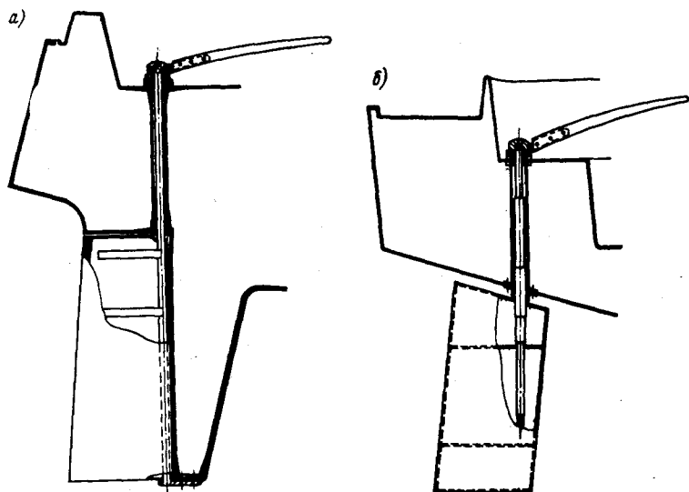
Рис. 129. Конструкции рулевого устройства на пластмассовой яхте.
