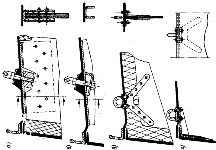
Рис. 137. Схема установки вант-путенсов.
