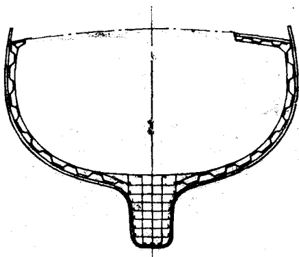
Рис. 112. Конструкция рамного шпангоута. Слева — для деревянной палубы, справа — для палубы из армоцемента.
