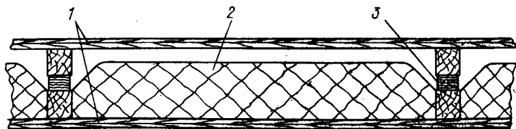
Рис. 148. Легкая переборка с шумопоглощающей изоляцией. 1 — фанера; 2 — шумопоглощающая изоляция; 3 — резиновая прокладка.
