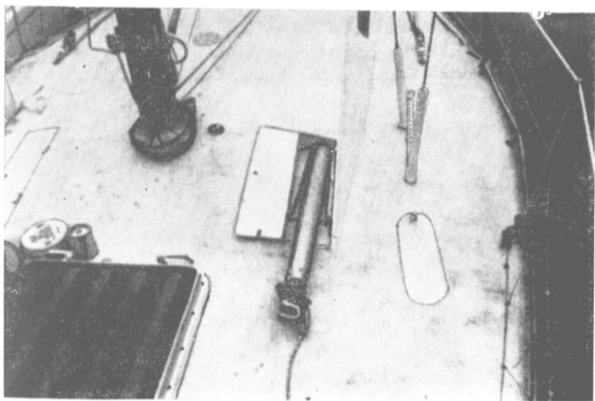
Рис. 165. Труба для хранения спиннакер-гика по-походному, вмонтированная в палубу.
