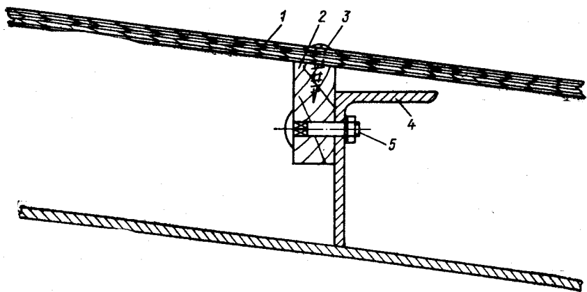
Рис. 149. Узел крепления внутренней зашивки к набору.
