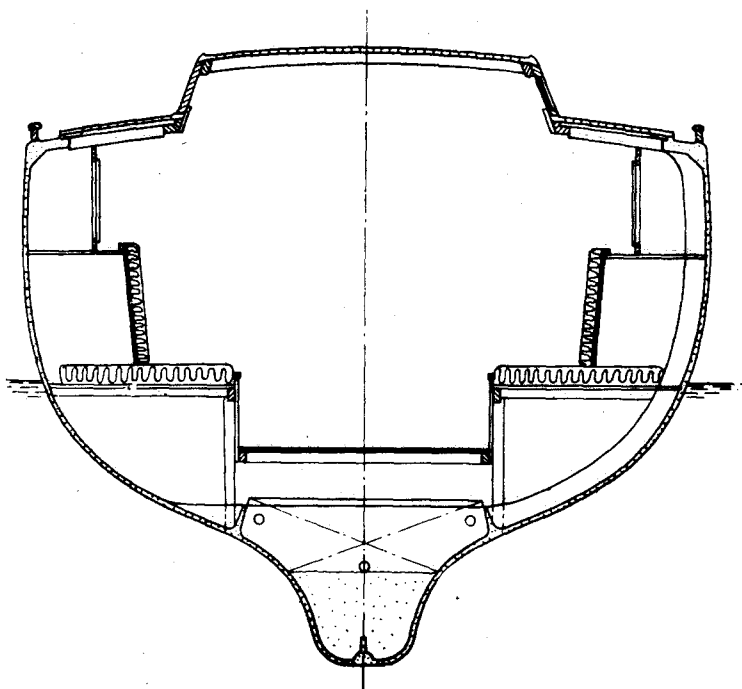
Рис. 108. «Мидель-шпангоут» 12-метрового крейсерского кэча из армоцемента.
