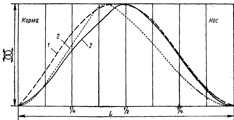
Рис. 8. Типичные строевые по шпангоутам различных яхт.
