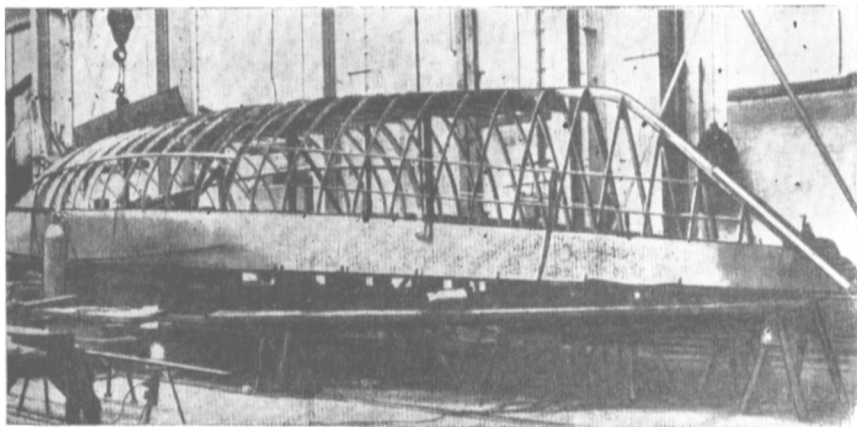
Рис. 93. Сборка корпуса в положении килем вверх на палубе. Обшивать корпус начинают с ширстрека.
