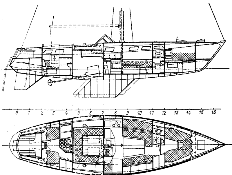
Рис. 58. Схема общего расположения «Гидры».
