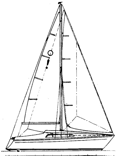
Рис. 30. Яхта «Омега-S» с баком элегантнее, просторнее, немного легче и благодаря надстройке является абсолютно остойчивой.
