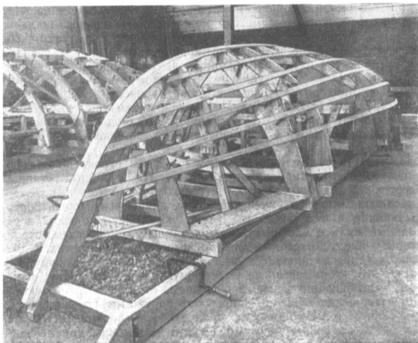
Рис. 73. Сборка корпуса с продольной системой набора.
