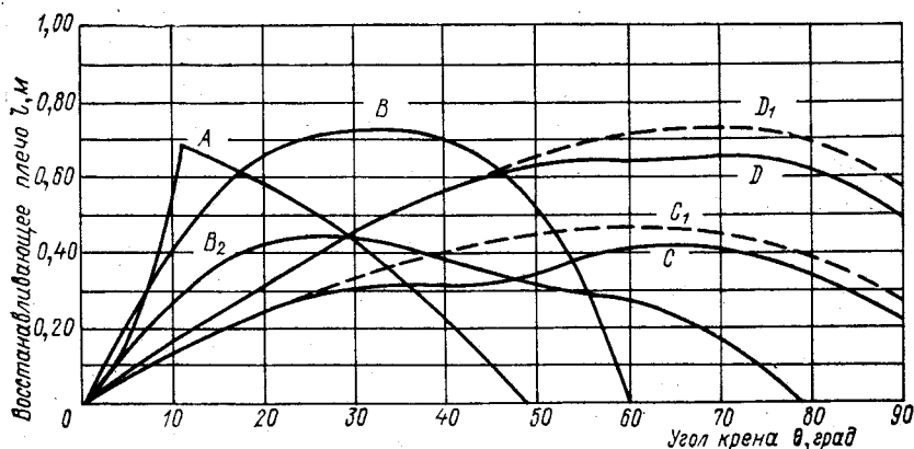
Рис. 1. Типичные диаграммы статической остойчивости.
