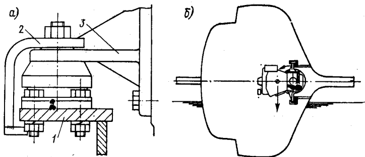
Рис. 177. Ограничитель амортизатора (а) и схема для расчета прочности крепления двигателя к фундаменту (б).
