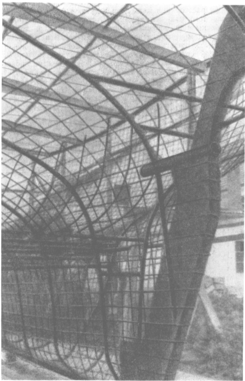
Рис. 114. Конструкция ахтерштевня, сваренного из стали, с закрепленной на наборе сеткой.
