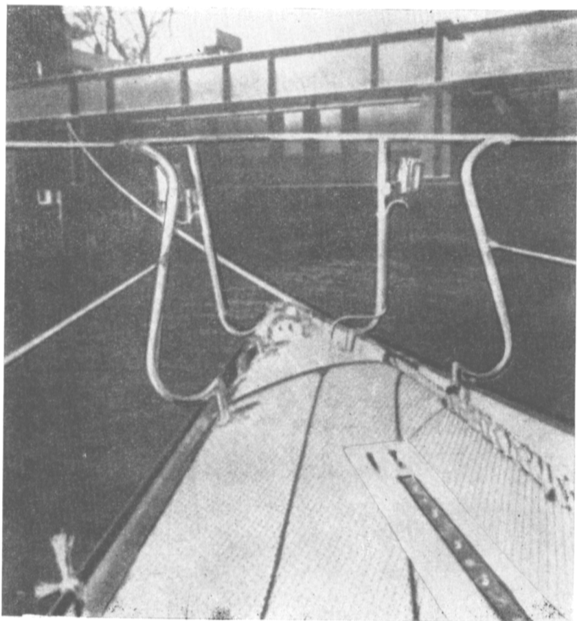
Рис. 166. Носовой реллинг, приспособленный для крепления по-походному двух спинакер-гиков.
