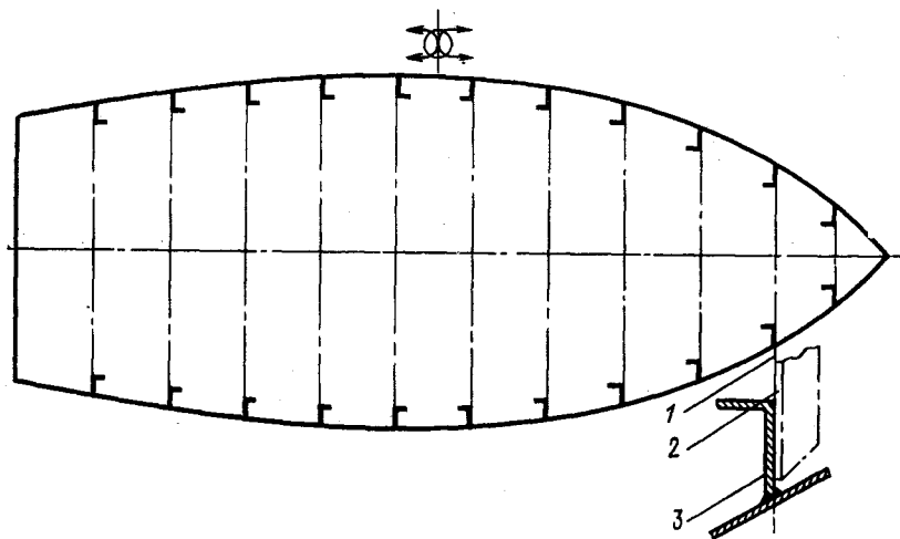
Рис. 91. Теоретические линии и направление полкок шпангоутов в металлическом корпусе.
