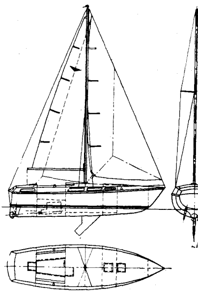
Рис. 24. Проект глиссирующей моторно-парусной яхты с узким корпусом (ширина ограничена по условиям транспортировки).
