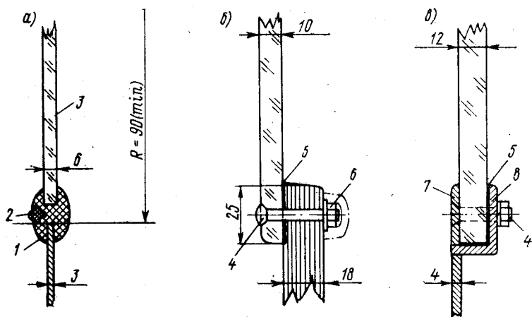
Рис. 150. Типовое исполнение неподвижных (глухих) иллюминаторов: а — с использованием резинового обжимного профиля, заимствованного из автомобилестроения; б — крепление съемного иллюминатора из акрилового стекла на винтах; в — вставной иллюминатор в металлической раме.
