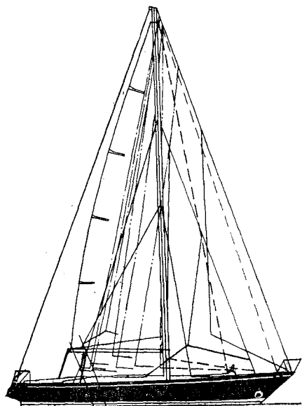
Рис. 43. Схема парусности яхты «Саудад».
