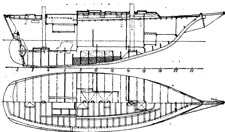
Рис. 109. Конструктивный чертеж кэча из армоцемента.
