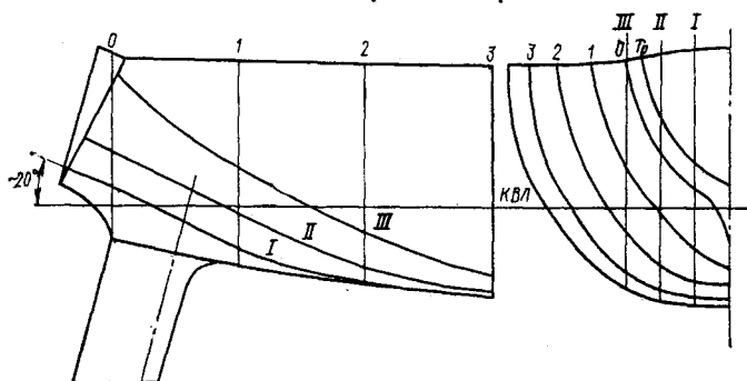
Рис. 11. Плоская корма водоизмещающего судна с углом выхода батоксов до 20^\circ . Желательна концентрация водоизмещения в корме, необходимая для достижения сверхкритической скорости.
