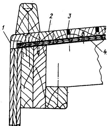
Рис. 67. Типовая конструкция настила палубы из фанеры, поверх которой наклеены планки из тика (расстояние между палубными бимсами 300—400 мм).
