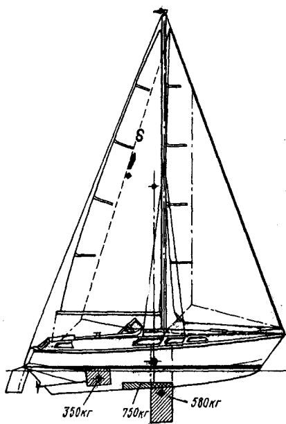
Рис. 20. Остойчивость яхты «Секура» с подъемным килем может быть рассчитана на случай убранного кия точно так же, как для нормального плавания с опущенным килем. Дополнительный внутренний балласт обеспечивает абсолютную остойчивость и при поднятом выдвижном киле.
