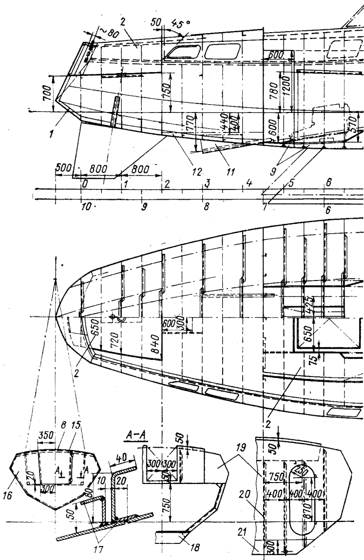
Рис. 5. Конструктивный чертеж корпуса 14-метровой яхты «Гидра».
