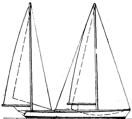
Рис. 169. Оригинальное парусное вооружение (двойной шлюп) яхты «Ондин» конструкции Бриттона Ченса.
