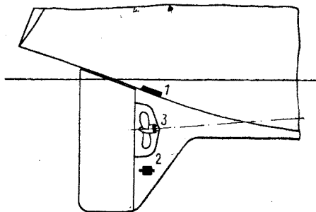
Рис. 203. Расположение защитных анодов на алюминиевой яхте.
