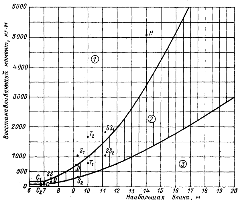
Рис. 21. Зависимость остойчивости яхты от их длины и района плавания. 1 — яхты неограниченного района плавания (категории 1 и 2); 2 — яхты морского плавания (категории 3 и 4); 3 — яхты с ограниченной остойчивостью (немореходные яхты).
