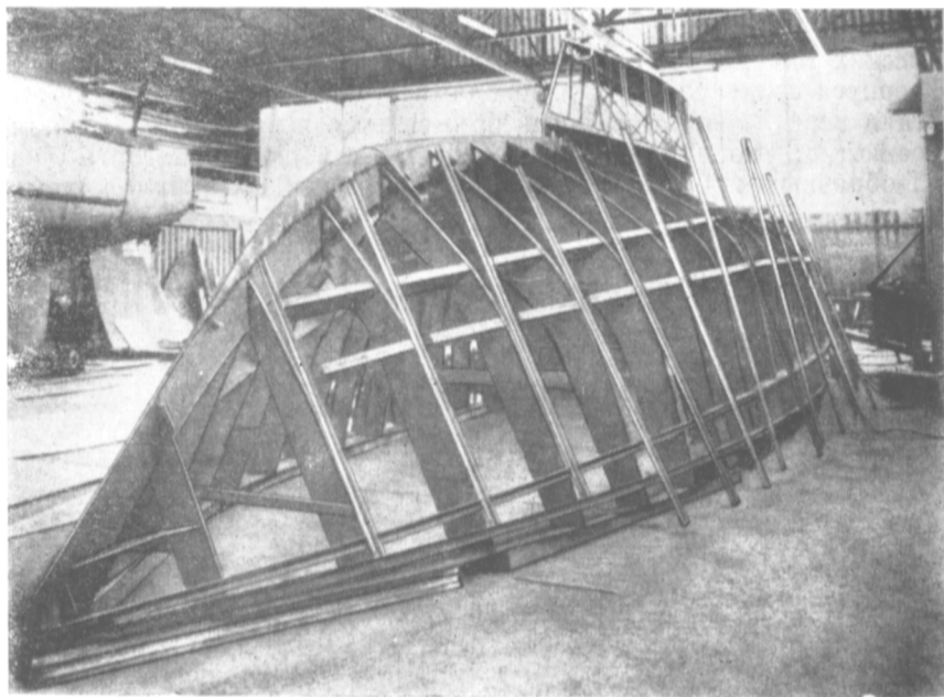
Рис. 94. Гамбургская верфь «Фельтц» строит серийные корпуса из стали, используя относительно недорогое приспособление. Благодаря гибке поперечных шпангоутов на месте, не требуется заранее изготавливать шпангоутные рамы.
