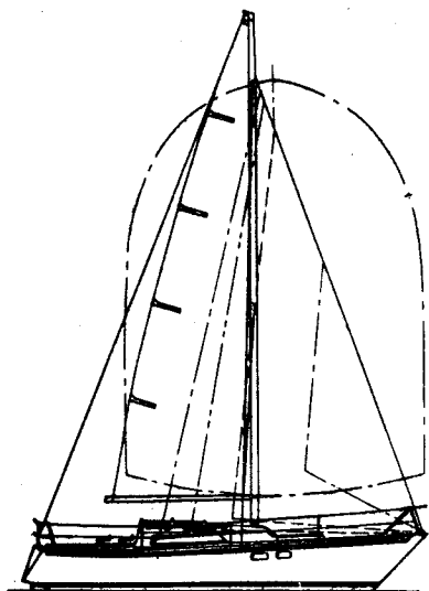
Рис. 26. Схема парусности яхты «Пион»: грот — 19 м 2 ; генуя № 1 — 28,9 м 2 ; генуя № 2 — 24,7 м 2 ; стаксель № 1 — 18,6 м 2 ; стаксель № 2 — 12,5 м 2 ; штормовой стаксель — 6,4 м 2 ; толбой — 12,1 м 2 ; спинакер — 62 м 2 ; ричер — 29,1 м 2 .
