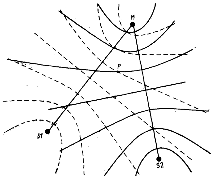
Рис. 193. Упрощенное изображение сети гипербол системы «Лоран». Множество гипербол образуется основной станцией M и двумя вспомогательными S_1 и S_2 . Местонахождение судна P определяется точкой пересечения линий положения двух пар передатчиков.
