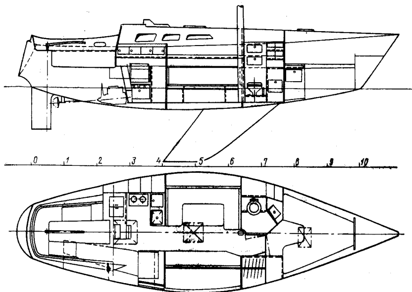
Рис. 35. Схема общего расположения яхты «Ченс-32/28».
