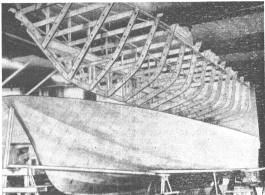
Рис. 70. Остов-шаблон освобожден от склеенной оболочки корпуса.
