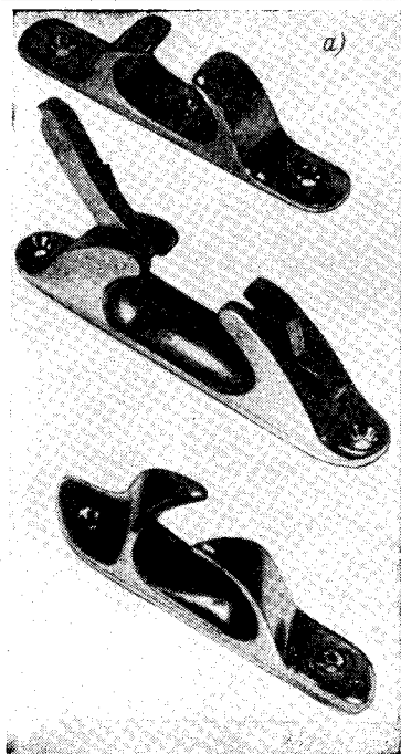
Рис. 154. Дельные вещи швартовного устройства: а — киповые планки (полуклюзы); б — утка и кнехты.
