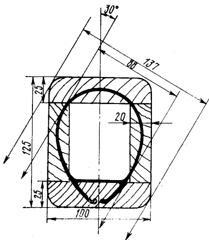
Рис. 153. Мачта яхты «Омега» из дерева и алюминия.
