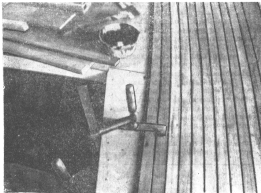
Рис. 68. Давление для склеивания тиковых планок, где это возможно, создают с помощью струбцины.
