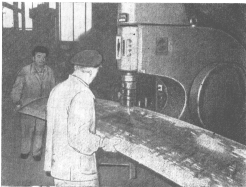
Рис. 86. Благодаря тому что края листов под прессом сокращаются, листам наружной обшивки придадут продольную погибь и одновременно усиливают поперечную погибь.
