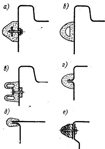
Рис. 126. Крепление привальных брусьев к корпусу.
