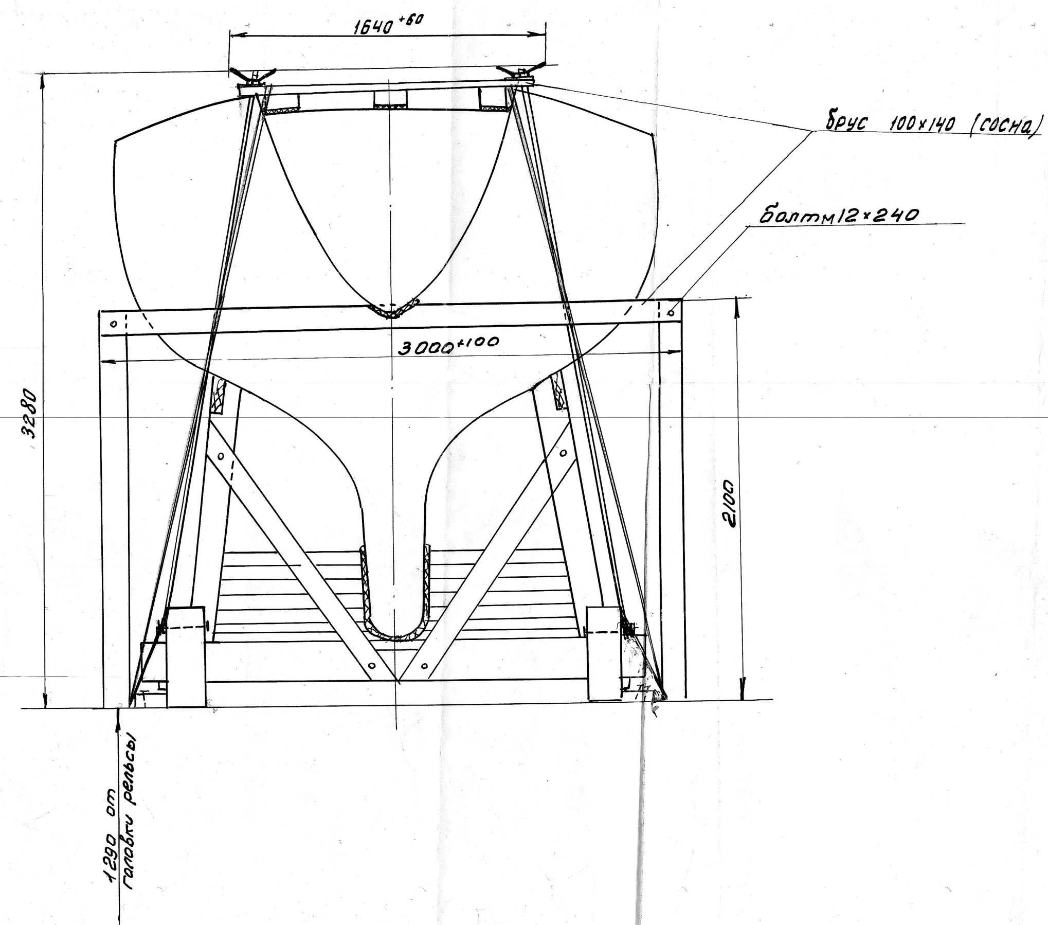
Разрез В-В
