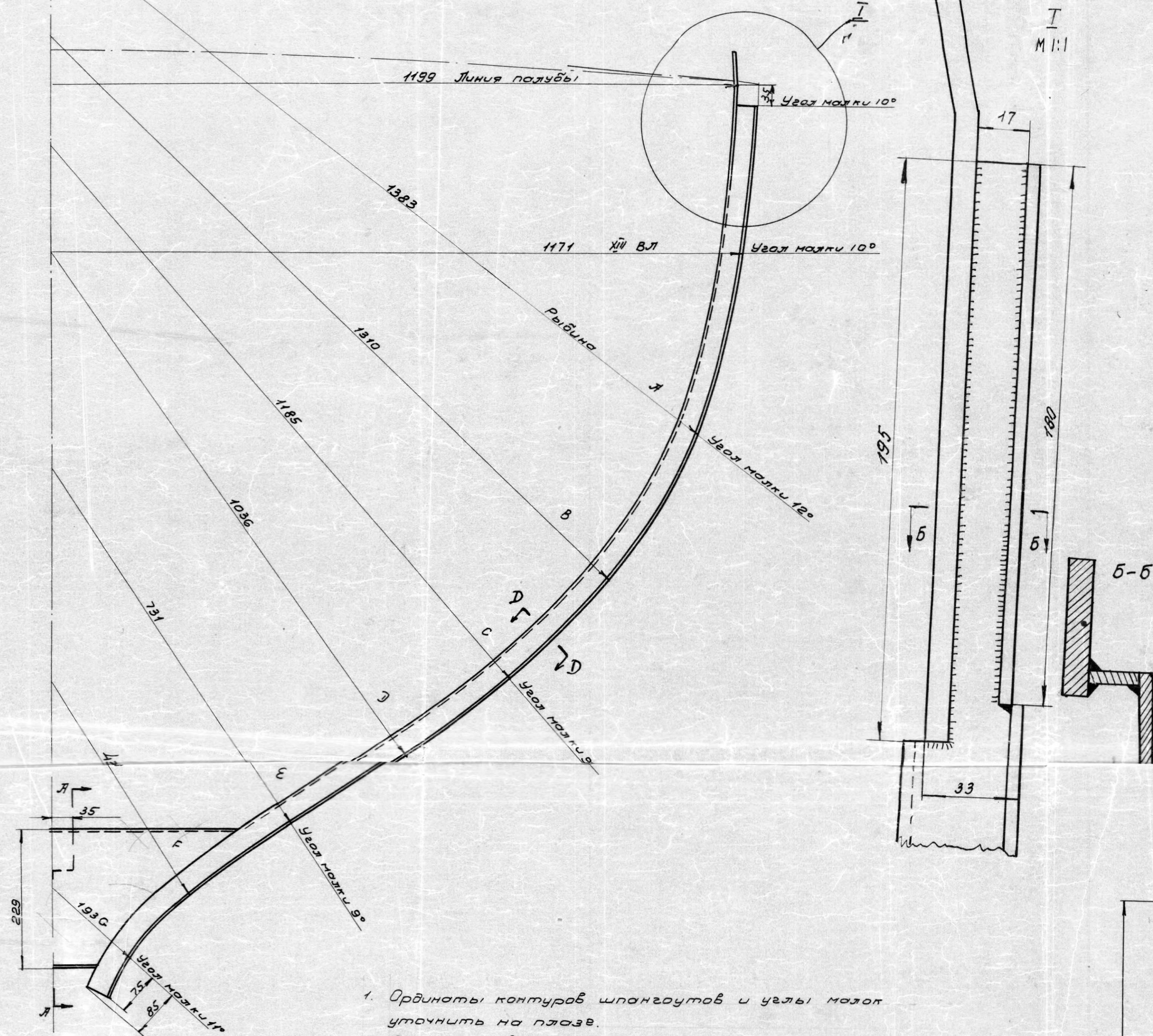
Шпангоут №25 М1:5
