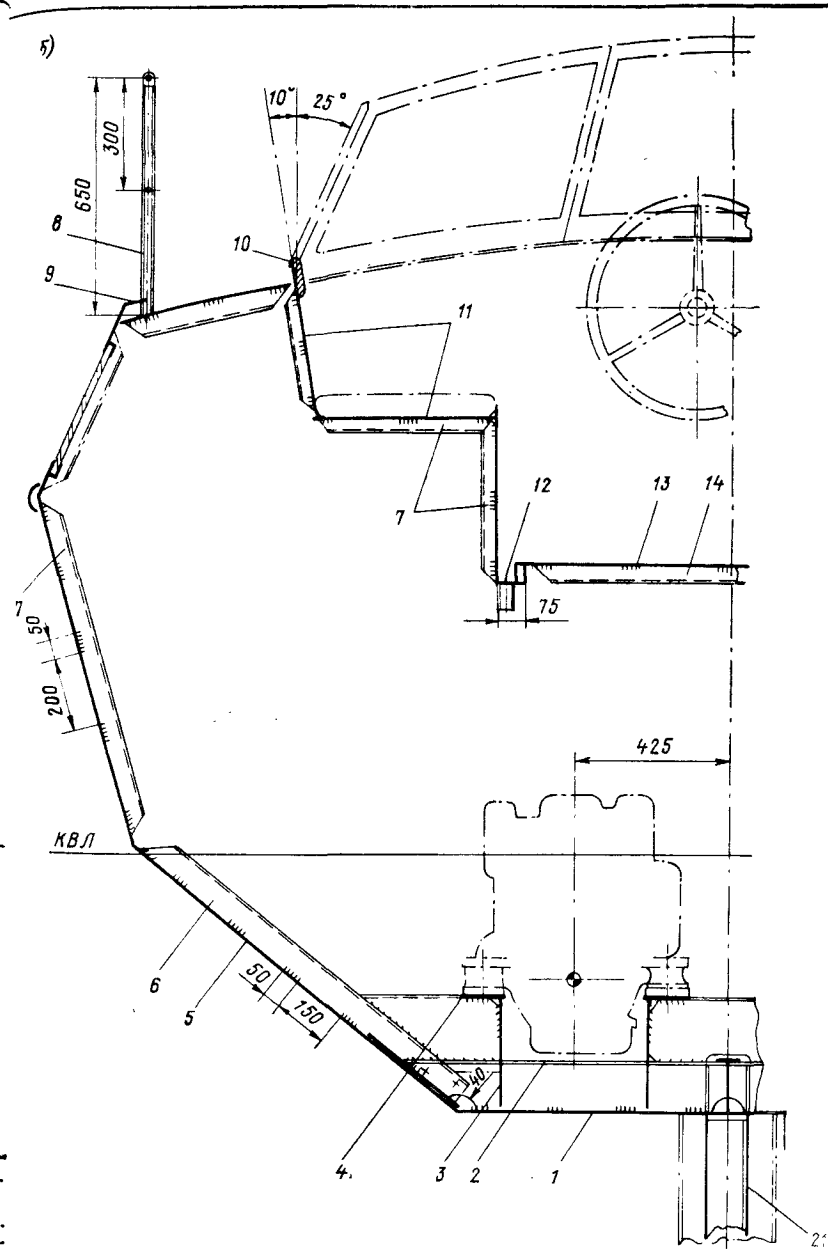
Рис. 4, а, б. Конструктивный «мидель-шпангоут» стальной яхты «Гидра»: а — сечение по шп. 3/4, см. рис. 5; б — сечение по шп. 6/7, см. в нос; [В скобках указаны толщины для корпуса из легкого сплава].
