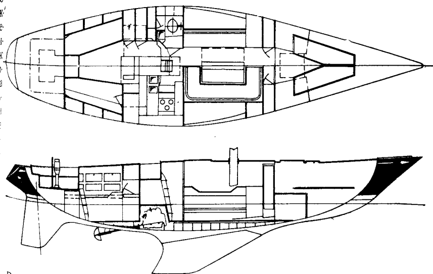
Рис. 42. Схема общего расположения яхты «Саудад».
