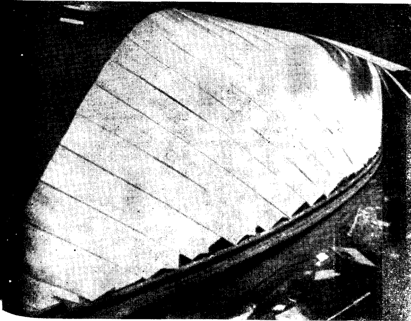
Рис. 79. Подогнанные и прихваченные скобами листы шпона надо снимать по отдельности и после нанесения клея вновь укладывать на болван.
