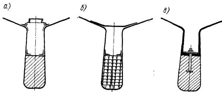
Рис. 130. Балластные кили.
