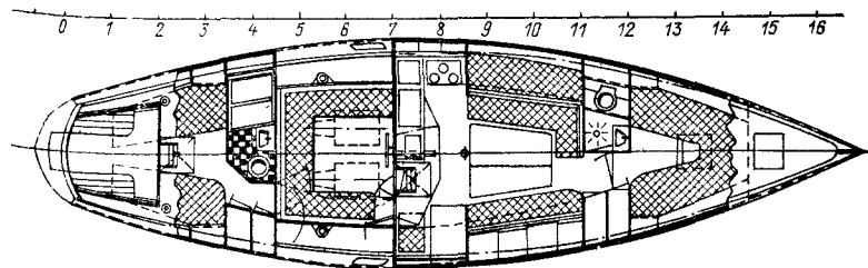
Рис. 58. Схема общего расположения «Гидры».
