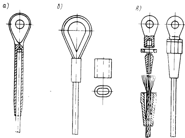
Рис. 162. Наконечники для тросов стоячего такелажа: а — наконечник, напрессовываемый на трос; б — втулка, напрессованная на трос, согнутый в петлю; в — разъемный наконечник типа «Норсман».
