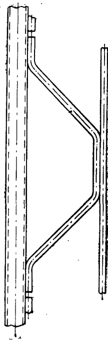
Рис. 114. Конструкция ахтерштевня, сваренного из стали, с закрепленной на нем сеткой.
