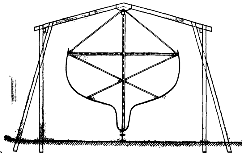
Рис. 110. Поперечное сечение стапеля.
