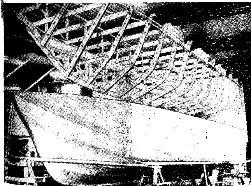
Рис. 70. Остов-шаблон освобожден от склеенной оболочки корпуса.
