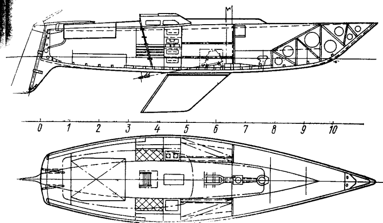
Рис. 48. Схема общего расположения яхты «Импробэйбл».
