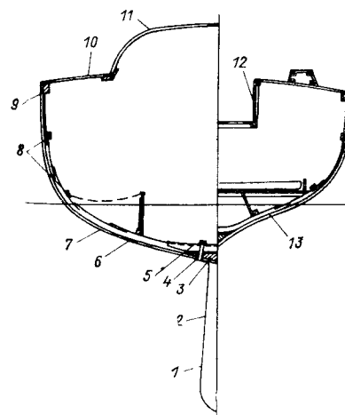
Рис. 49. Конструктивный мидель-шпангоут «Импробэйбл».
