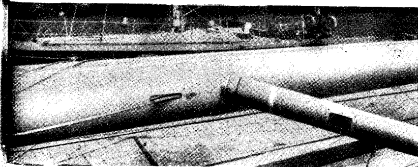
Рис. 160. Крепление основных вант и краспиц на алюминиевой мачте крейсера-гонимой яхты.
