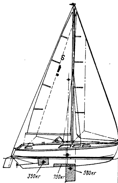
Рис. 20. Остойчивость яхты «Секур» с подъемным килем может быть рассчитана на случай убранного килем, точно так же, как для нормальной плавания с опущенным килем. Дополнительный внутренний балласт обеспечивает абсолютную остойчивость и при поднятом выдвижном киле.
