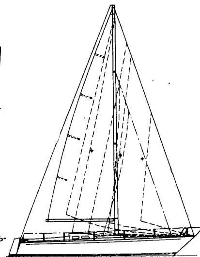
Рис. 50. Схема парусности «Импробэйбл».
