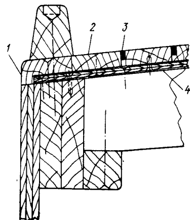
Рис. 67. Типовая конструкция настила палубы из фанеры, поверх которой наклеены планки из тика (расстояние между палубными бимсами 300—400 мм). 1—ватервейс 40×18, тик; 2—планка 40×12, тик; 3—пал, заполненный резиновым клеем, 8×4; 4—фанера, 6—6.
