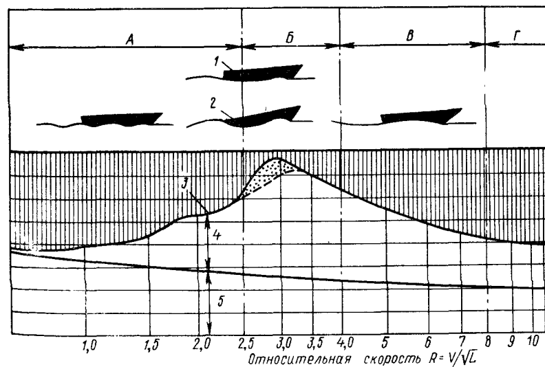
Рис. 7. Режимы движения яхты и зависимость сопротивления трения и формы от относительной скорости судна. V — скорость, уз; L — длина по КВЛ, м; A — водоизмещающее плавание; B — переходный к глиссированию режим; V — полуглиссирование; \Gamma — чистое глиссирование. 1 — современные обводы яхты; 2 — традиционные обводы яхты; 3 — кривая сопротивления; 4 — сопротивление формы; 5 — сопротивление трения.
