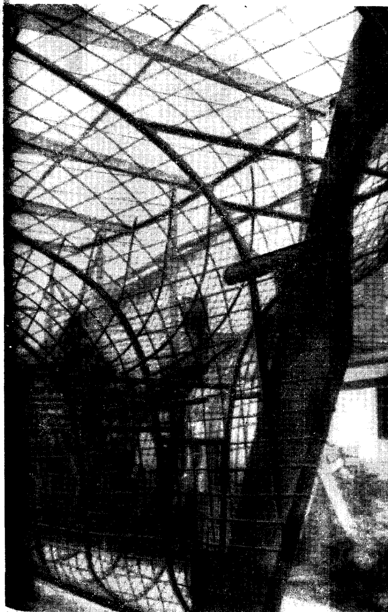
Рис. 114. Конструкция ахтерштевня, сваренного из стали, с закрепленной на нем сеткой.
