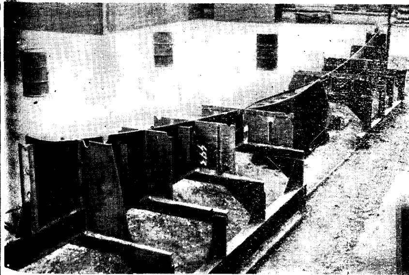
Рис. 102. Для постройки стапеля на неровном полу не обойтись без нескольких бетонных опор. В середине стапеля виден установленный киль, который в этом месте заменяет стапель.
