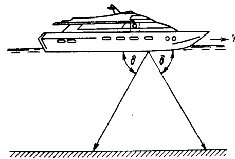
Рис. 197. Принцип лага Допплера: вибратор излучает ультразвуковые волны, направленные вперед и назад. Из сравнения частоты приема и передачи можно измерить двойное смещение и тем самым скорость судна.
