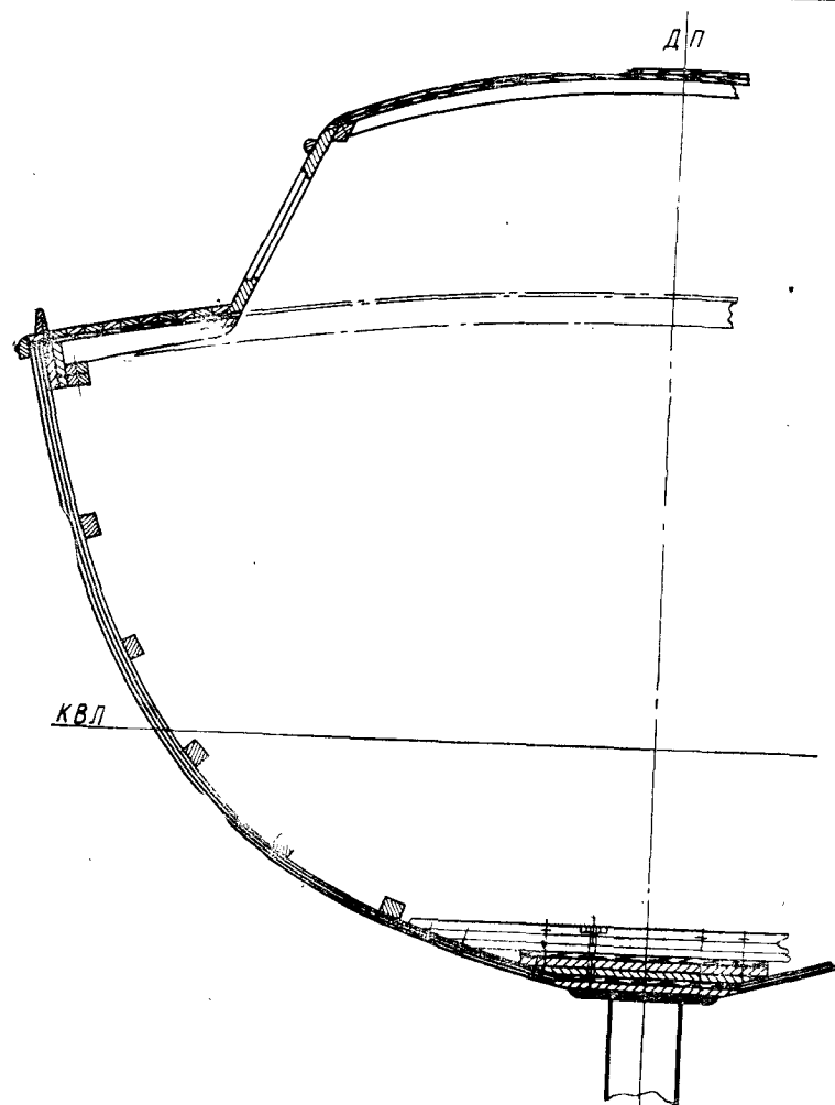
Рис. 75. «Мидель-шпангоут» яхты «Дести-С» длиной 9,20 м с наружной обшивкой из трех слоев судостроительной фанеры толщиной по 5 мм.
