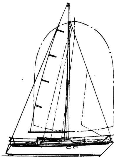
Рис. 26. Схема парусности яхты «Пион»: грот — 19 м 2 ; генуя № 1 — 28,9 м 2 ; генуя № 2 — 24,7 м 2 ; стаксель № 1 — 18,6 м 2 ; стаксель № 2 — 12,5 м 2 ; штормовой стаксель — 6,4 м 2 ; толлбол — 12,1 м 2 ; спинакер — 62 м 2 ; рич — 29,1 м 2 .
