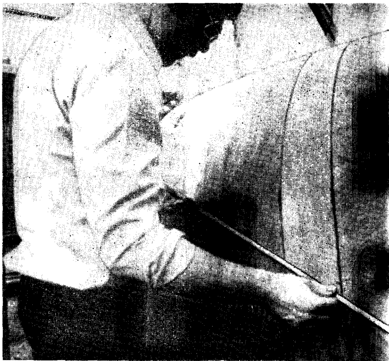
Рис. 77. Диагональная обшивка из полос фанеры на стпель-кондукторе
