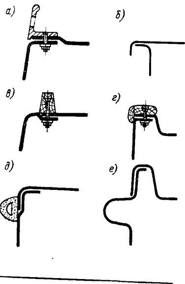
Рис. 125. Узлы соединения палубы с корпусом.
