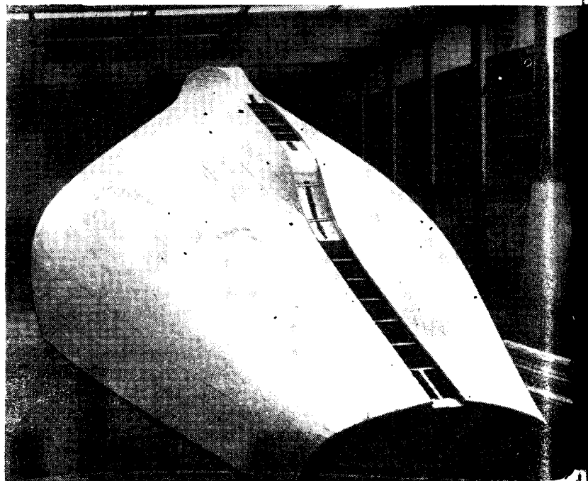
Рис. 78 Болван — положительная форма, на которой строят клееные корпуса. Он стоит примерно в два раза дороже, чем построенный по нему корпус.
