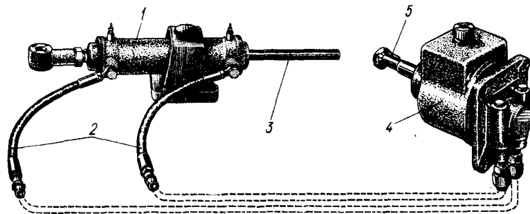
Рис. 142. Ручное гидравлическое рулевое устройство (50—1600 Н·м). 1—гидравлический цилиндр двойного действия; 2—гибкие трубопроводы; 3—рулевой сектор; 4—гидронасос; 5—вал рулевого колеса.
