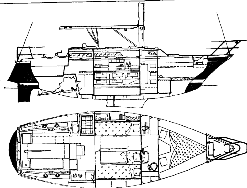
Рис. 44. Схема общего расположения яхты «Дюфур-31».
