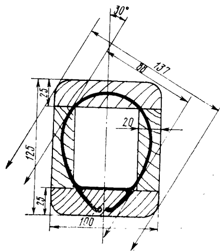
Рис. 159. Мачта яхты «Омега» из дерева и алюминия.
