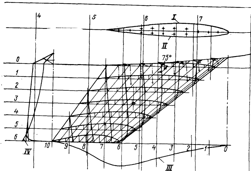
Рис. 15. Теоретический чертеж плавникового киля.
