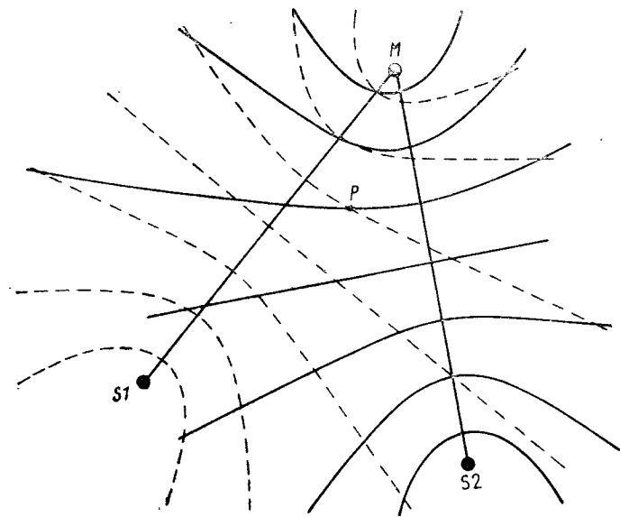
Рис. 193. Упрощенное изображение сети гипербол системы «Лоран». Множество гипербол образуется основной станцией M и двумя вспомогательными S1 и S2 . Местонахождение судна P определяется точкой пересечения линий положения двух пар передатчиков.
