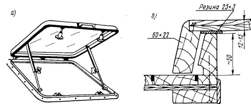
Рис. 152. Конструкция входных люков: а — люк из алюминия и акрилового стекла с минимальным комингсом и резиновым уплотнением; б — деревянный люк с комингсом, образующим водопоток.
