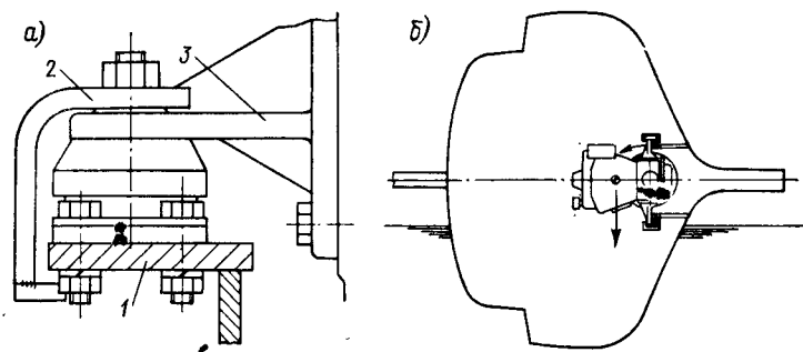
Рис. 177. Ограничитель амортизатора (а) и схема для расчета прочности крепления двигателя к фундаменту (б). 1 — опорная плита фундамента; 2 — ограничитель; 3 — лопастной двигатель.
