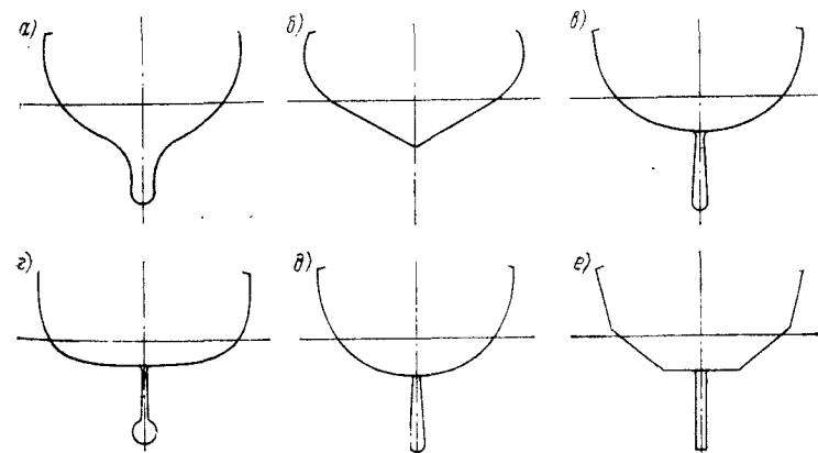
Рис. 6. Типичные обводы шпангоутов яхт: а — S -образный; б — V -образный; в — радиальный; г — U -образный; д — шпангоут трапецеидальный; е — шпангоут с двойной скулой.
