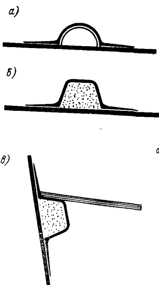
Рис. 127. Конструкции стрингеров.
