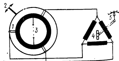
Рис. 200. Принцип телепередачи направления ветра на индикатор (сельси).
