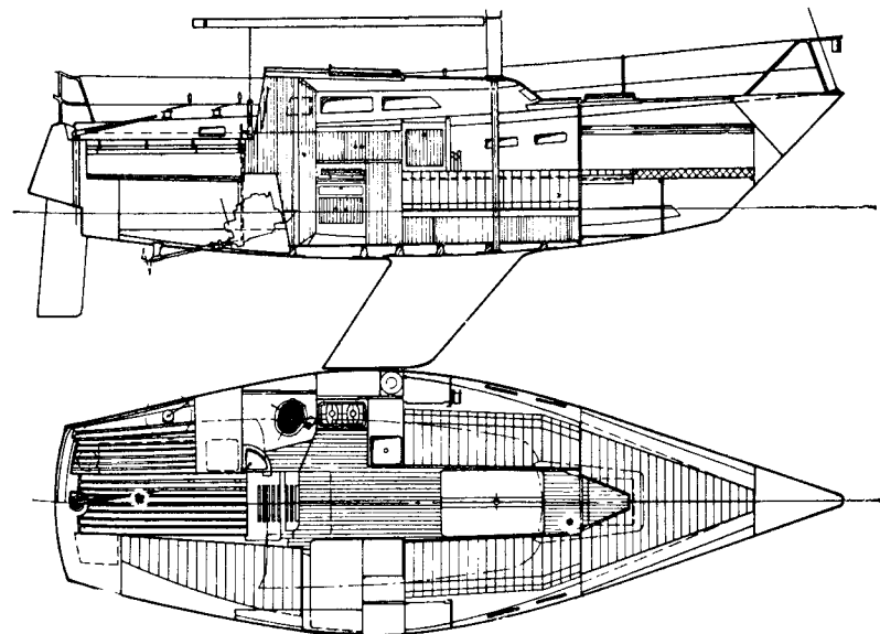
Рис. 25. Общее расположение яхты-моно типа «Пион». Основные данные: наибольшая длина 9,05 м; длина по КВЛ 7,10 м; ширина 2,93 м; осадка 1,66 м, водоизмещение 3,80 т. Балласт 1,53 т. Площадь парусности около 38 м 2 .
