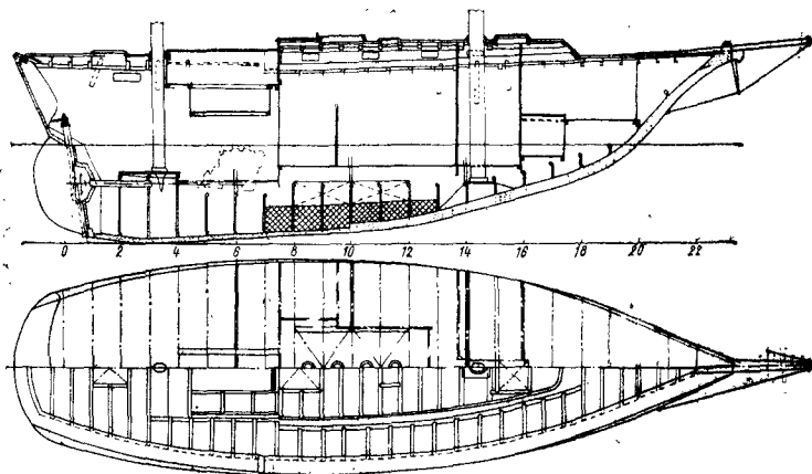
Рис. 109. Конструктивный чертеж кэча из армоцемента.
